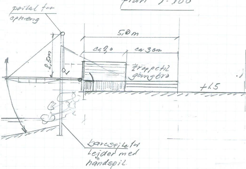
opstalt 1:100
