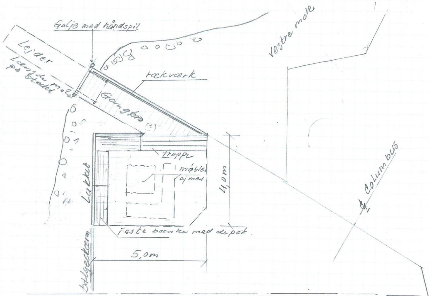
plan 1:100
