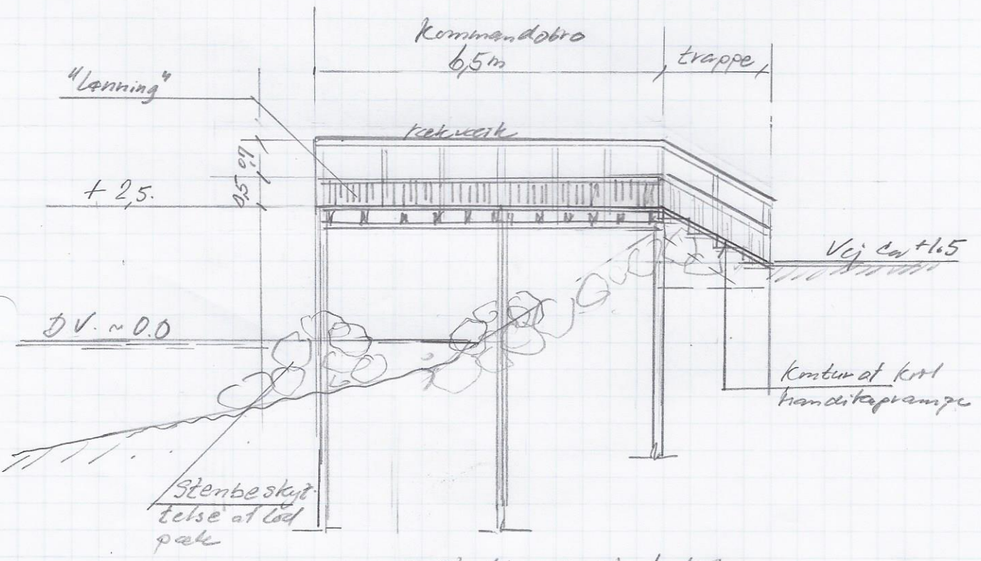
opstalt - snit 1:100
